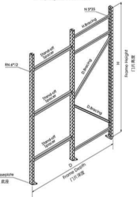
โครงสร้าง 3 เสา 3 Uprights Frame
