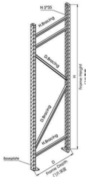
โครงสร้าง 2 เสา 2 Uprights Frame
